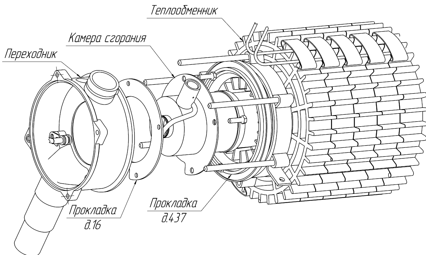
Рис.15–Схема установки КС в AIR-8D.
