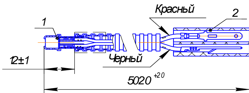
Рис. 18 – Датчик кабинный
