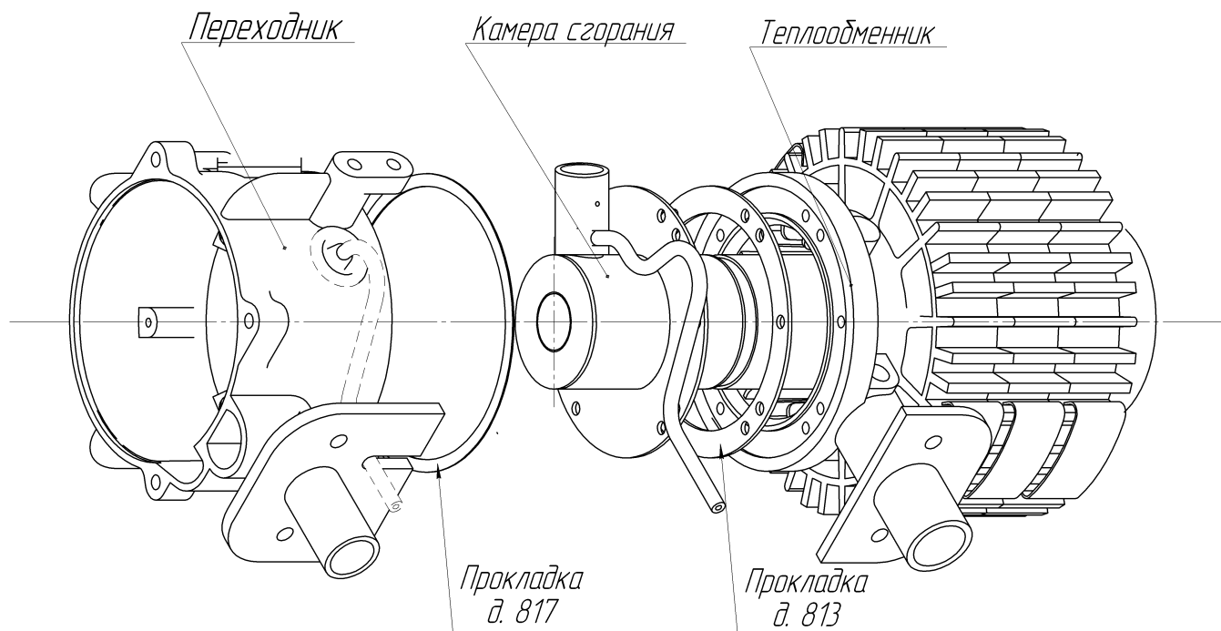
Рис.14–Схема установки КС в AIR-4D.
