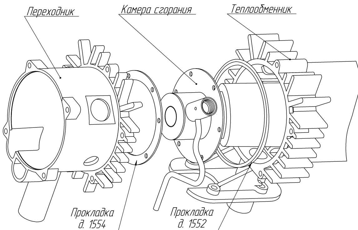
Рис.13–Схема установки КС в AIR-4D
