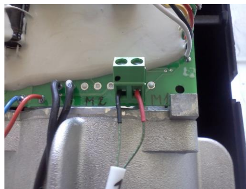
Рис. 9а – Подключение
