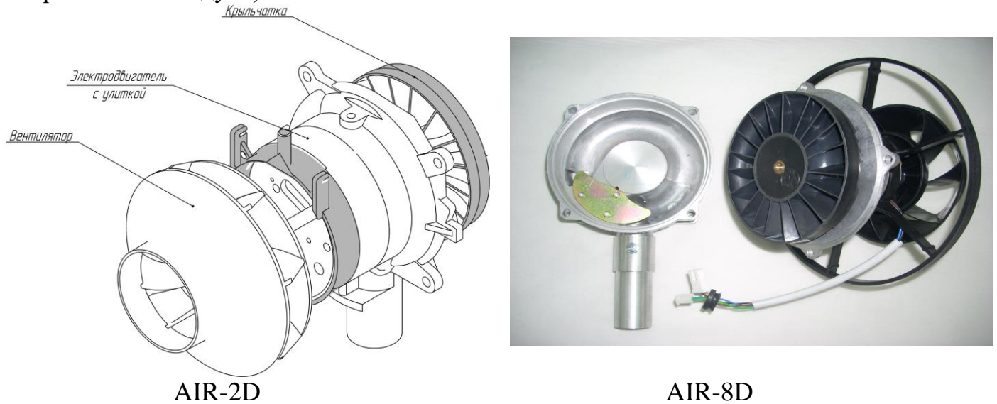
Рис.11 – Нагнетатель воздуха
